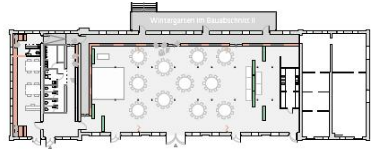
Grundriss 1:200
